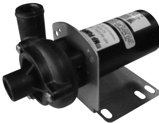
FRX 50-R
